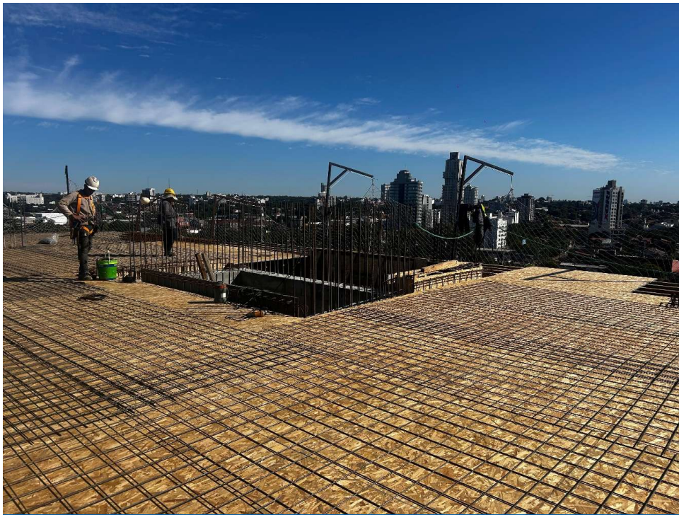
Trabajos de preparación de losa en Torre 21
