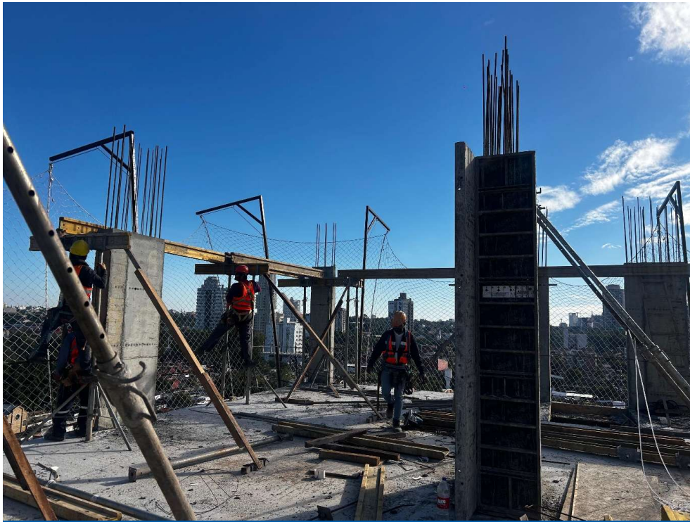
Trabajos de fondeo de losa y encofrado de pilares en Torre 20
