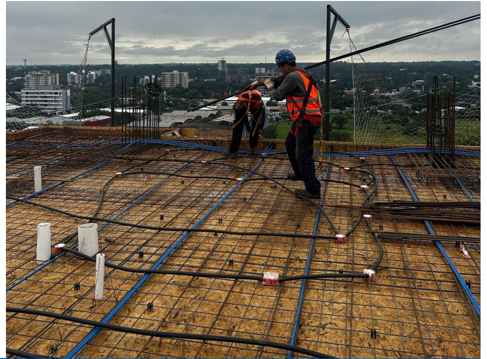
Trabajos de preparación de losa en Torre 21
